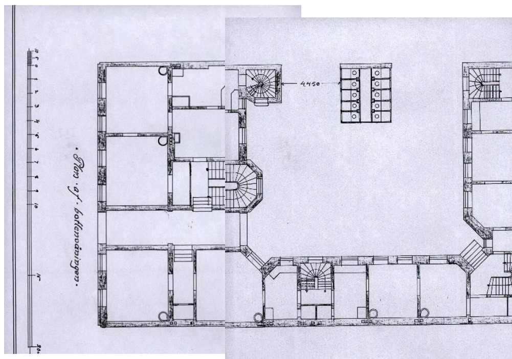
Bild 3. Delar av ritning över fastighetens bottenplan vid bygglovsansökan 1893.
